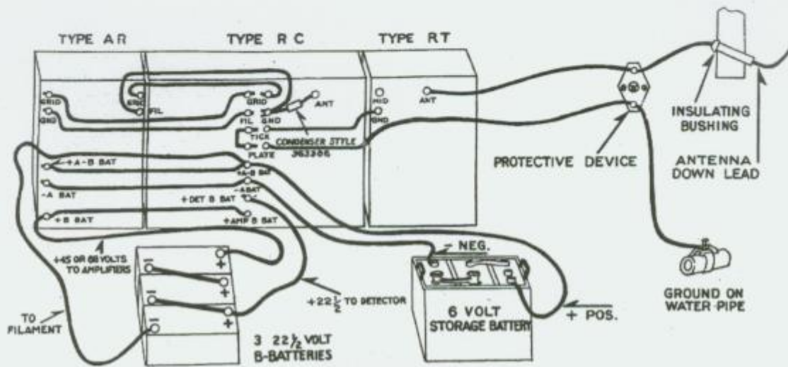
Fig. 3—Radiolas RT—RC—AR
